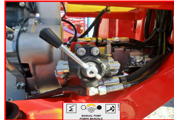
Afbeelding 61: kraan handpomp.
